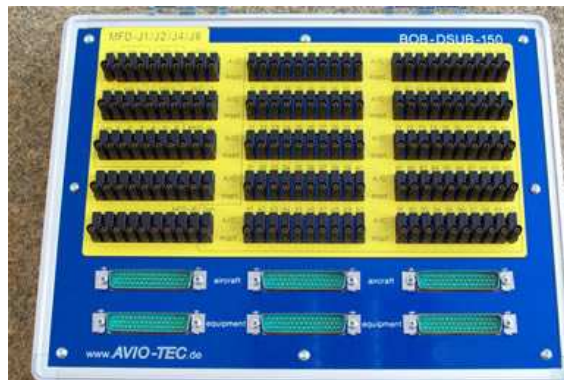
Break-out-Box mit Adapter bezogener Maske
